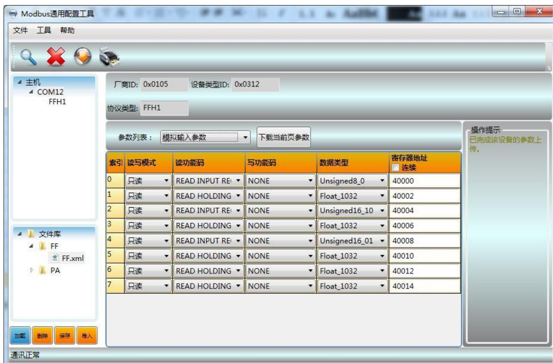
Figure 4.5 Parameter Configuration
